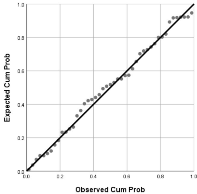
Fig. 1. Fisher p-plot chart
