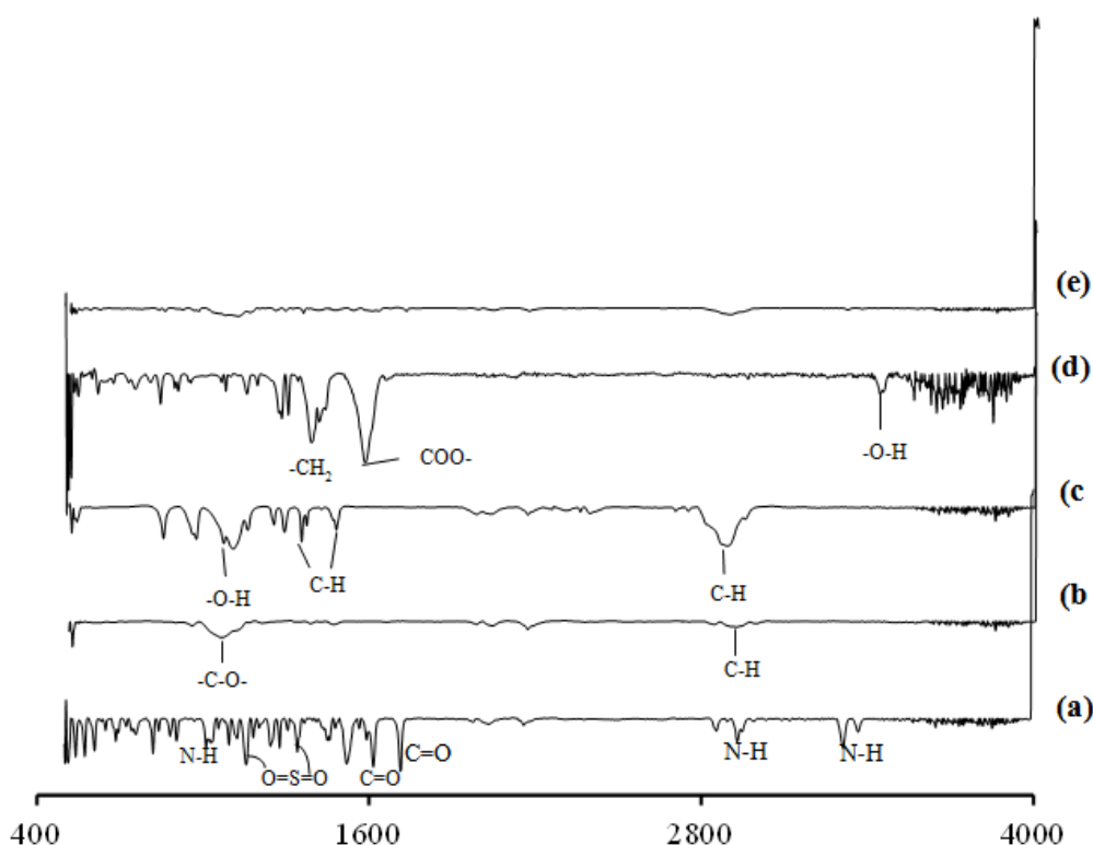
Fig. 4. FT-IR spectra of (a) GLB, (b) HPMC, (c) PEG-8000, (d) Na-citrate and (e) GCHP-4
